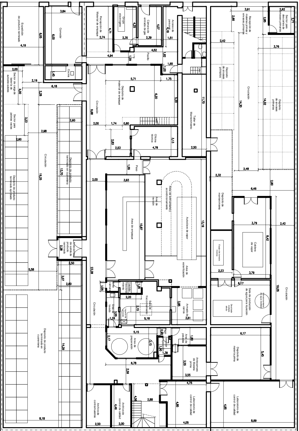
PLANTA BAJA
